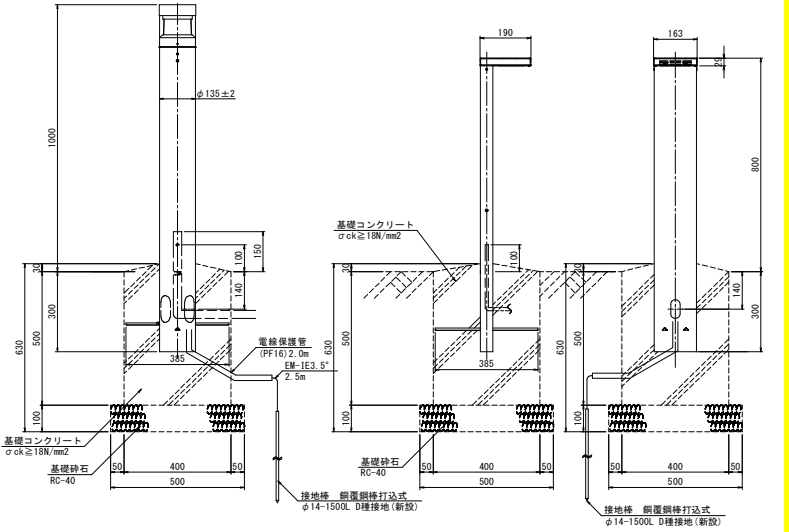
LEDランプ姿図 S=1:2 ランプ取替え
