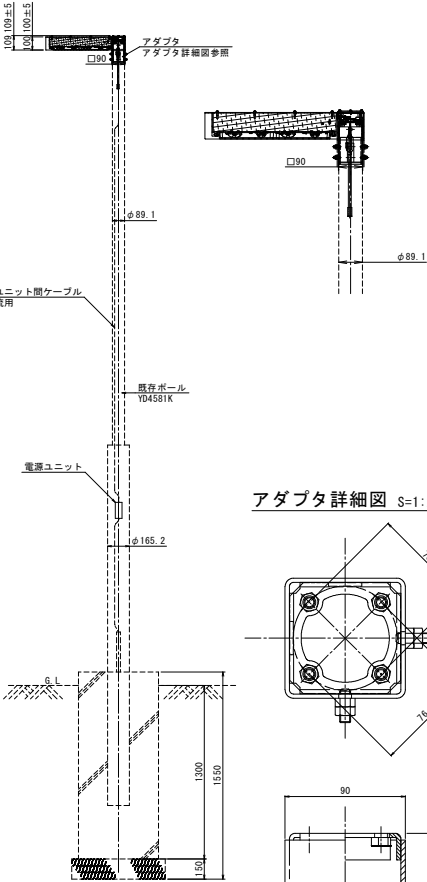
照明器具姿図 S=1:20 灯具のみ更新
