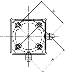
アダプタ詳細図 S=1:2
